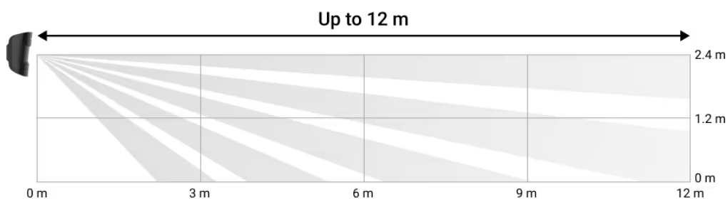
Angolo di visione verticale del rivelatore
