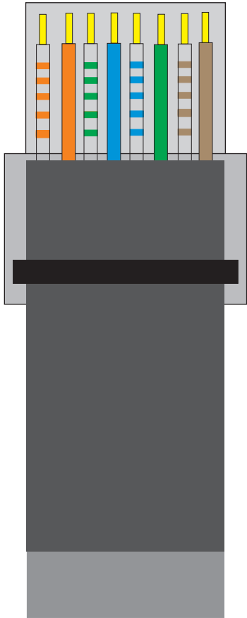
EIA/TIA 568B
